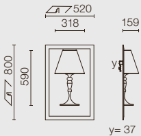
QT-32 max 75W
