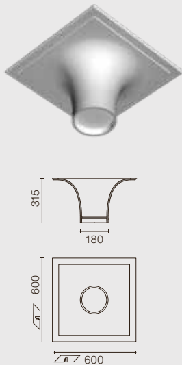
USO BOOB 600 1L
