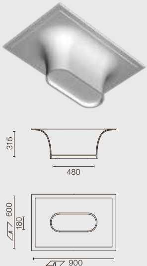
USO BOOB 600 2L
