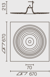
QR-CBC-51 max 50W
